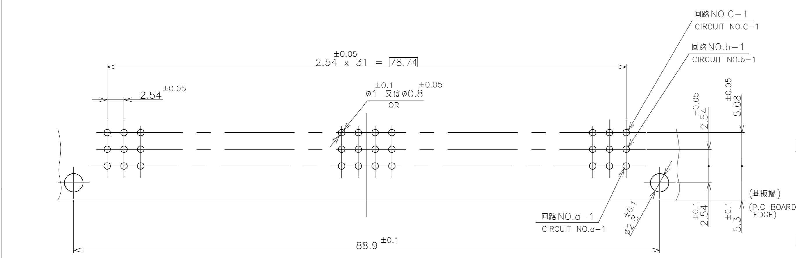
P.C. BOARD DIMENSIONS プリント基板 取付寸法 (コネクタ搭載面) (CONN. MOUNTING SIDE)
