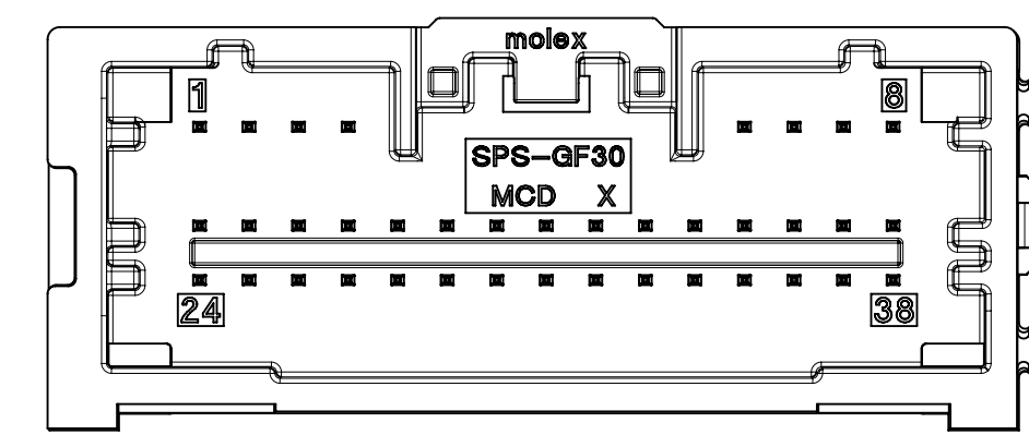
38WAY POLARIZATION UPDATED OPTION 'B' P/N: 34958-0384
